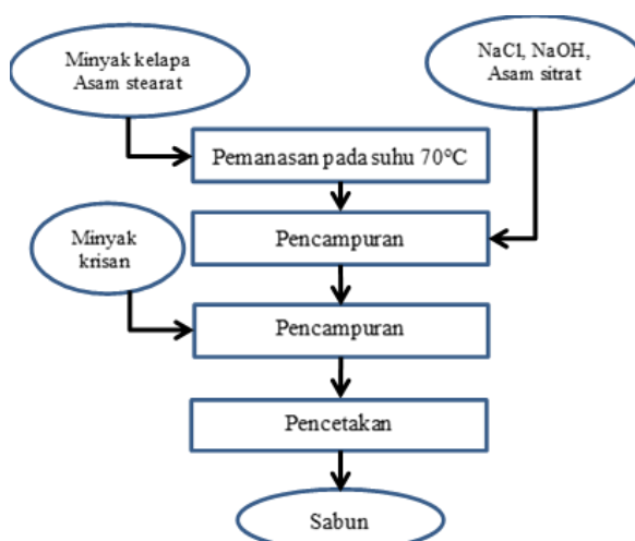
Gambar 6. Flow chart proses pembuatan sabun mandi padat dari minyak atsiri bunga krisan
