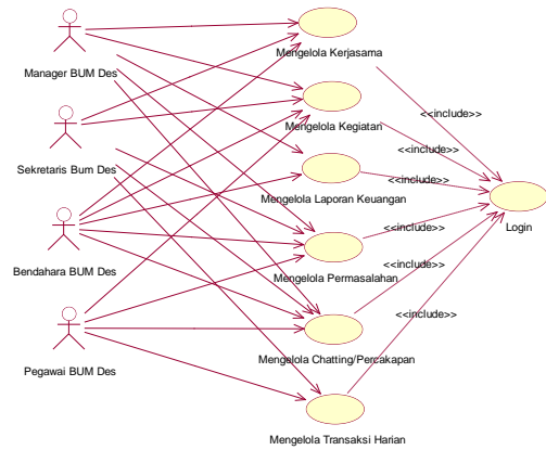
Gambar 3 Use case Aplikasi
