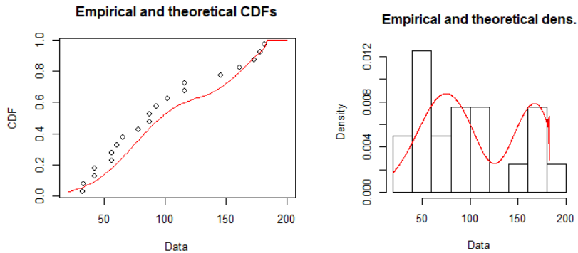
Gambar 3.1. Grafik estimasi cdf dan pdf distribusi WNL berdasarkan data
