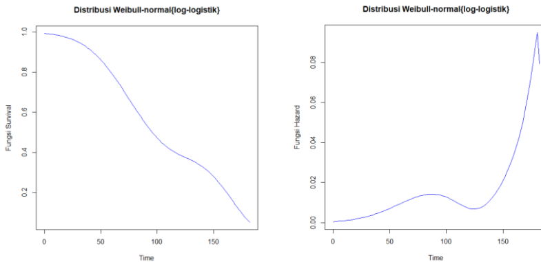
Gambar 3.2. Grafik estimasi fungsi survival dan fungsi Hazard distribusi WNL berdasarkan data
