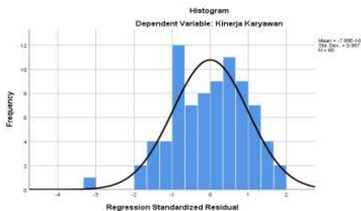
Gambar 1 Grafik Histogram
