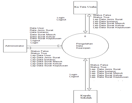
Gambar 3.1. Diagram Konteks
