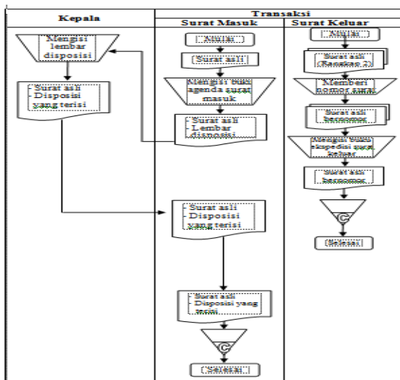
Gambar 1. Analisa Sistem Lama
