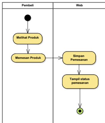
Sumber: Hasil Rancangan Penelitian Gbr. 2 Activity Diagram Pemesanan Produk
