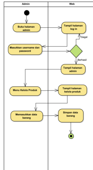
Sumber: Hasil Rancangan Penelitian Gbr. 3 Activity Diagram Pengelolaan Produk
