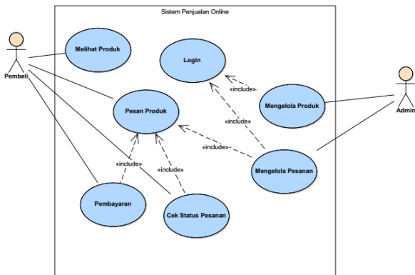
Sumber: Hasil Rancangan Penelitian Gbr. 1 Use Case Diagram Penjualan
