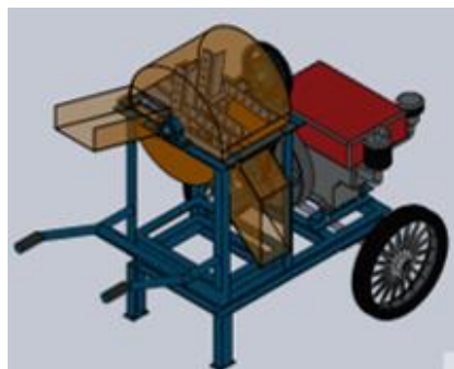
Gambar 2. Mesin Pencacah Pelepah Sawit Sistem Rotary
