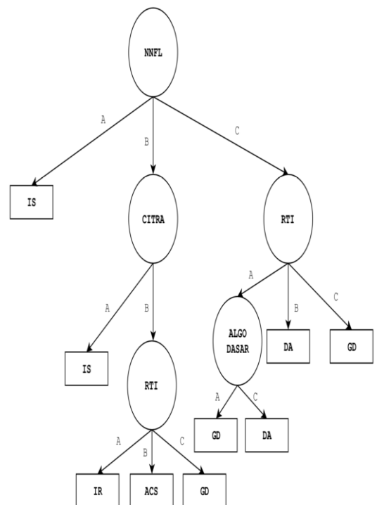
Gambar 2 Tree yang terbentuk
