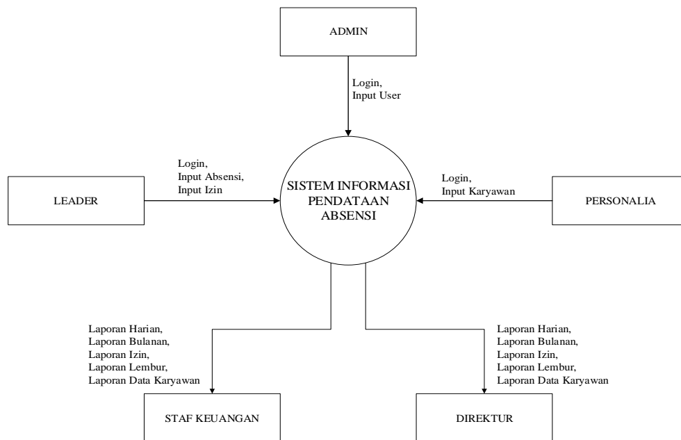
Gambar 1. Diagram Konteks Sistem usulan
