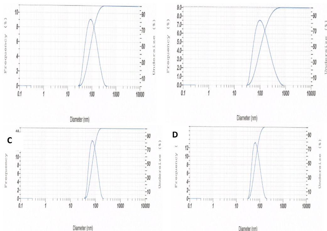
Gambar 6. Grafik Distribusi Ukuran Hasil Sintesis Nanopartikel Perak (A) pH 6, (B) pH 7, (C) pH 8, dan (D) pH 9
