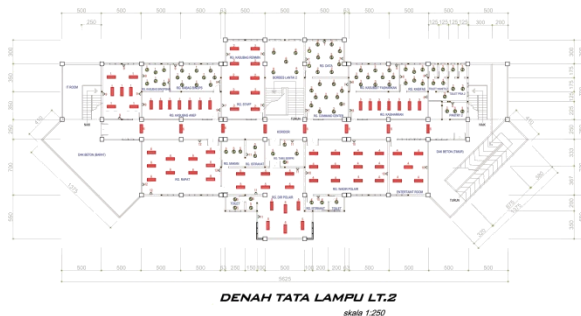
Gambar 2. Denah Gedung dan Tata Lampu Lantai 2
