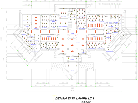
Gambar 1. Denah Gedung dan Tata Lampu Lantai 1
