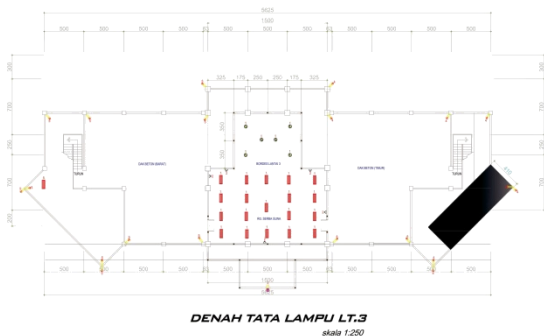
Gambar 3. Denah Gedung dan Tata Lampu Lantai 3
