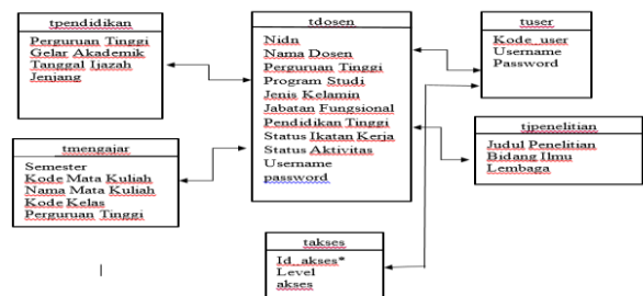
Gambar 5. Relasi Tabel
