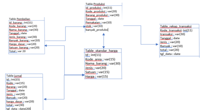
Gambar 4. Relasi Tabel
