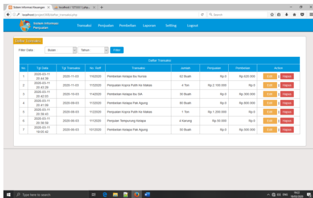
Gambar 7. Transaksi Penjualan
