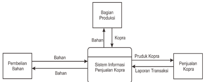
Gambar 3. Diagram Konteks
