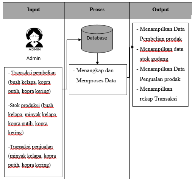
Gambar 1. Kerangka Sistem
