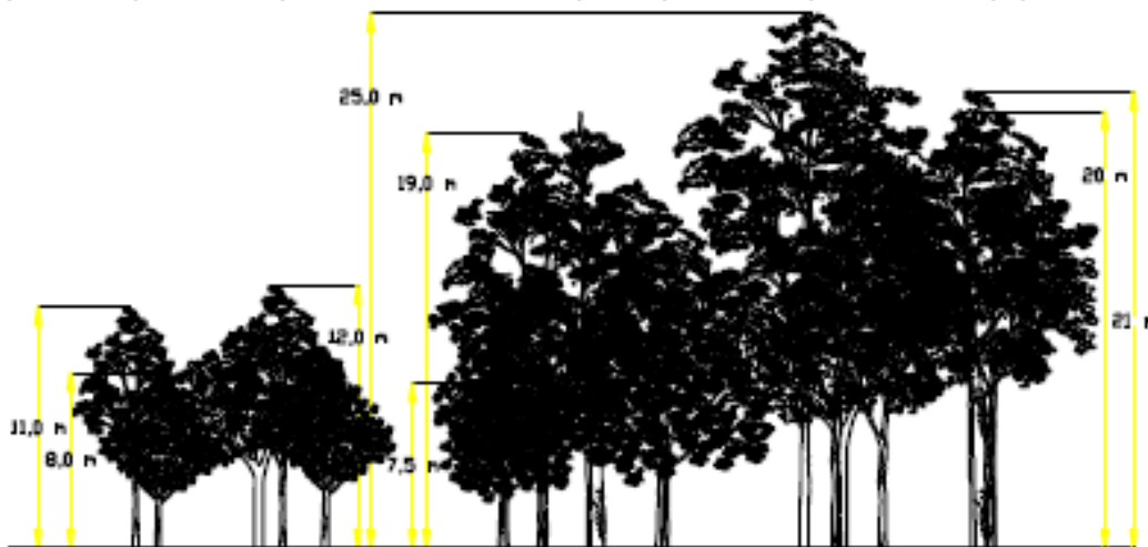
Gambar 1. Struktur Tegakan Vertikal (Diagram Profil) di Danau Baru
