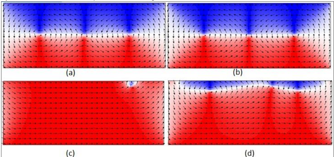
Gambar 4. Momen magnetik pada free layer (a) CoFeB ketika energi anisotropi bernilai maksimum dan (b) NiFe ketika energi anisotropi bernilai maksimum (c) NiFe ketika energi anisotropi medan magnet 20 mT (d) CoFeB ketika medan magnet 20 mT.
