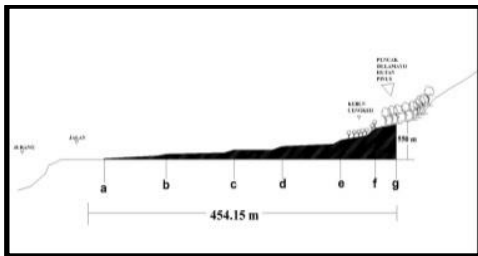
Gambar 3. Kontur Site Sumber: Data Analisa 2021
