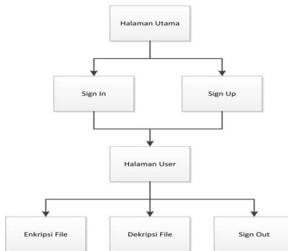
Gambar 7. HIPO Endesapp
