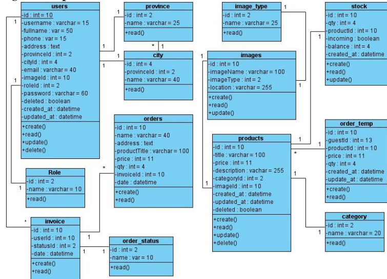
Gambar 3 Class Diagram Aplikasi M-Commerce
