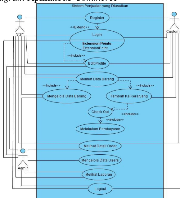
Gambar 2 Use Case Diagram Aplikasi M-Commerce
