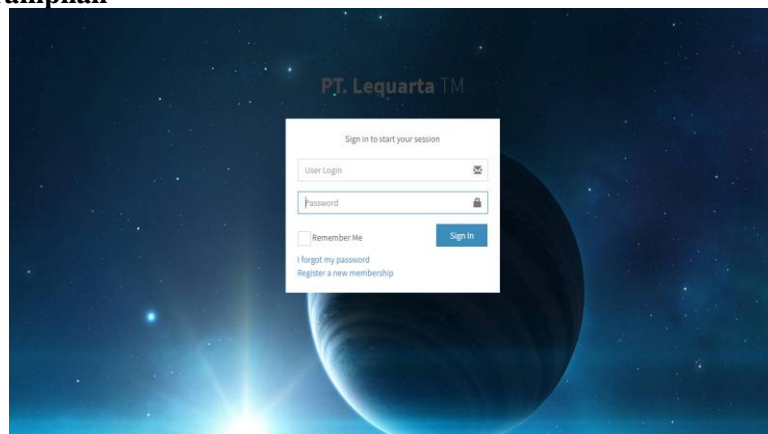
Gambar 6. Tampilan Login
