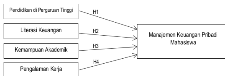
Gambar 1 Kerangka Penelitian
