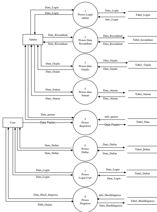
Gambar 3.2 DFD Level 1 Aplikasi Mengidentifikasi Jenis Kecanduan Akibat Penggunaan Narkotika dan Obat-obat Terlarang
