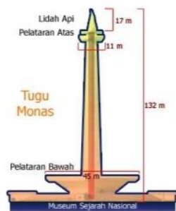
Gambar 7. Struktur Tugu Monas (sumber: https://id.wikipedia.org/wiki/Monumen_Nasional , 2017)
