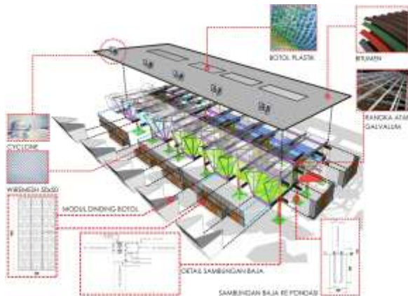
Gambar 23. Isometri bangunan
