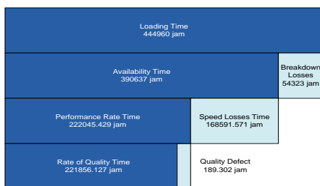
Gambar 5. Time Losses pada Mesin AMUT 1
