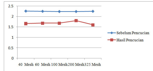
Gambar 1 Nilai Kadar Sulfur Batubara Setelah Pencucian
