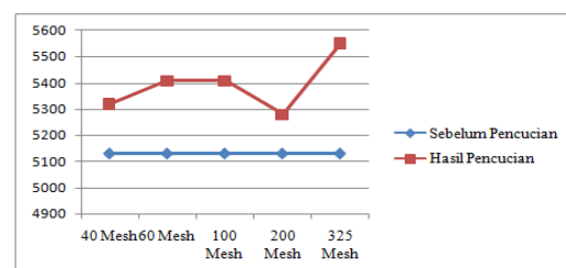
Gambar 2 Nilai Kalori Batubara Setelah Pencucian
