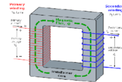
Gambar 1. Bagan Transformator
