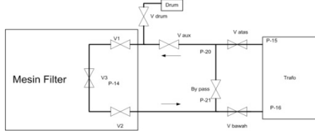
Gambar 2. Proses Filterisasi Internal Sumber: PT. PLN (PERSERO) P3B APP MALANG
