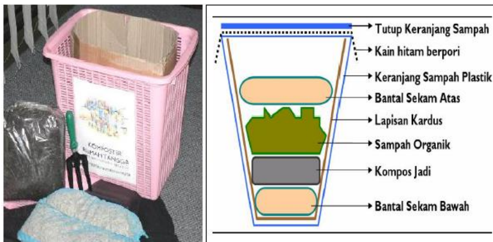
Gambar 1. Komposter Takakura
