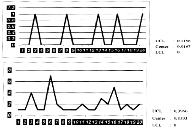
Gambar 4 Penurunan jumlah cacat dari sebelum dan sesudah perlakuan
