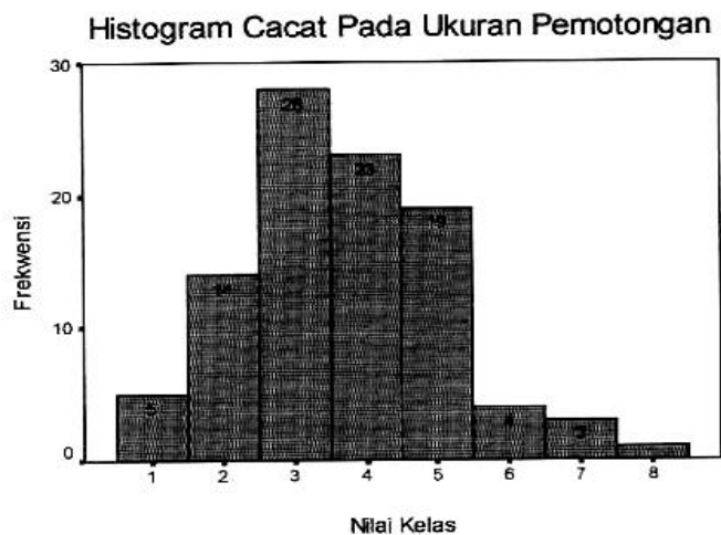
Gambar 3 Histogram cacat pada ukuran pemotongan
