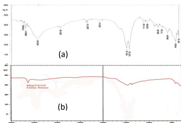
Gambar 4. (a) Spektra IR Mg(OH)_2 sampel dan (b) Spektra IR Mg(OH)_2 standar
