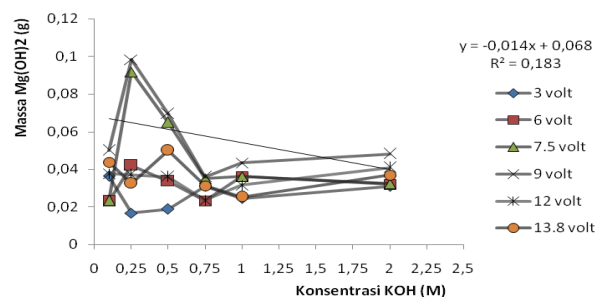
Gambar 3. Grafik pengaruh [KOH] terhadap perolehan massa Mg(OH) 2
