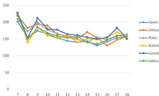
Gambar 6. Daya Luar Panel Surya
