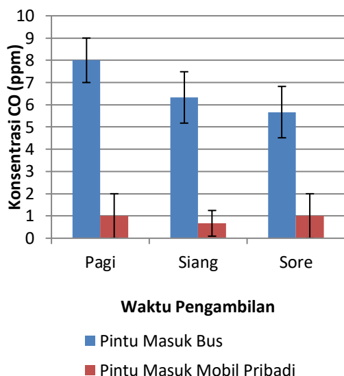
Gambar 3. Konsentrasi CO
