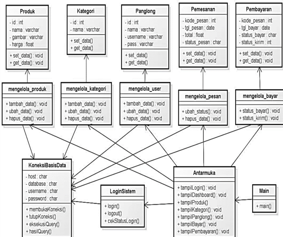
Gambar 2. Class Diagram Aplikasi Panglong
