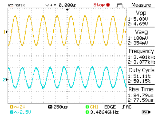
■ Gambar 11. Sinyal Pengukuran tanpa Filter
