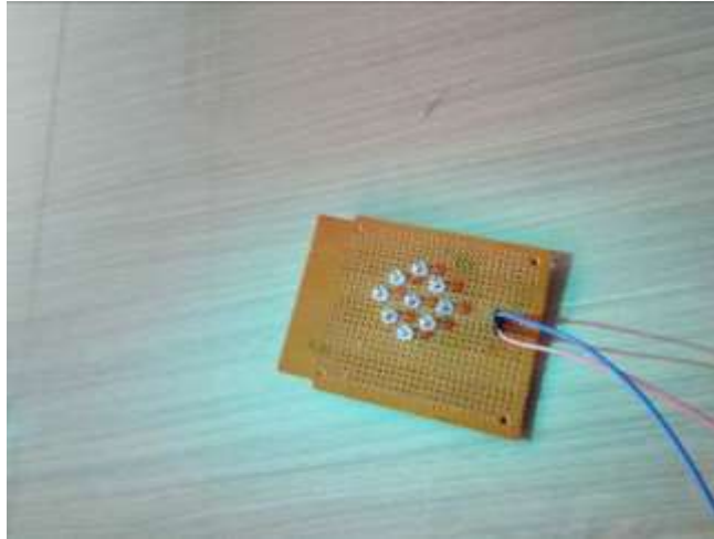
■ Gambar 19. Implementasi Pengukuran dengan Filter Warna Hijau
