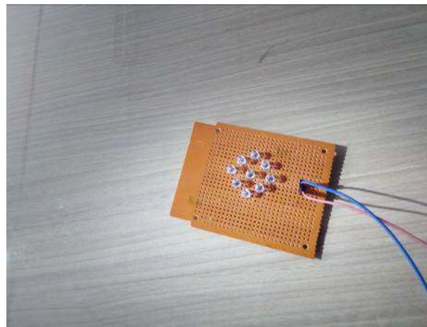
■ Gambar 16. Implementasi Pengukuran dengan Filter Warna Kuning
