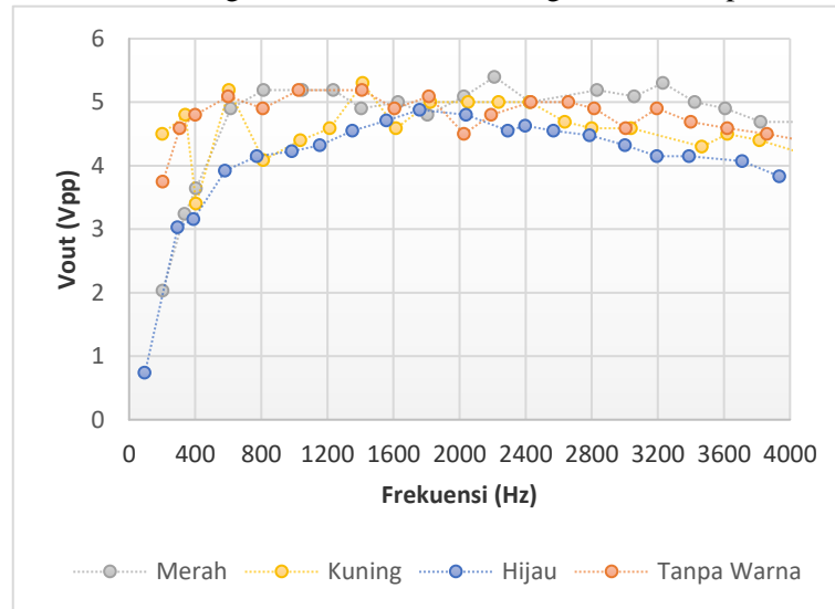
■ Gambar 22. Grafik Perbandingan Kualitas Penerima Sinyal.
