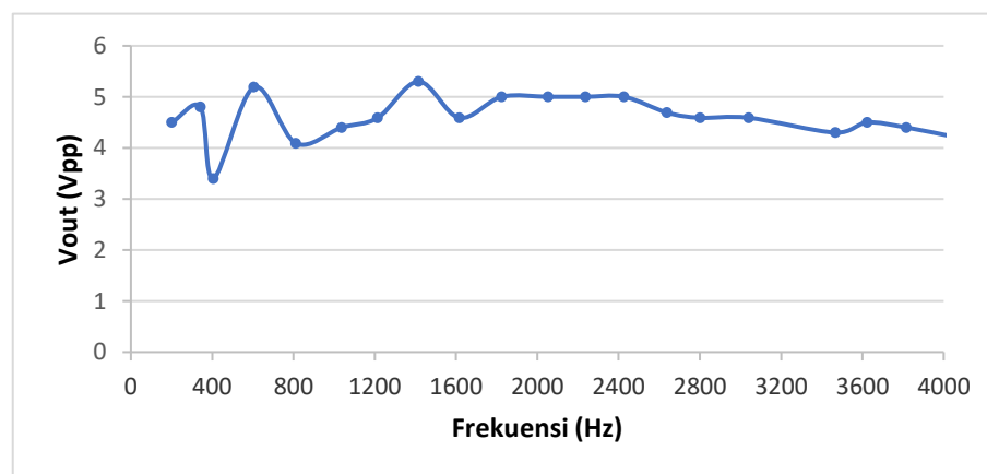
■ Gambar 18. Grafik Pengukuran dengan Filter Warna Kuning
