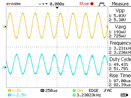
■ Gambar 13. Sinyal Pengukuran dengan Filter Warna Merah
