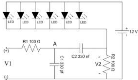
■ Gambar 6. Rangkaian Transmitter
