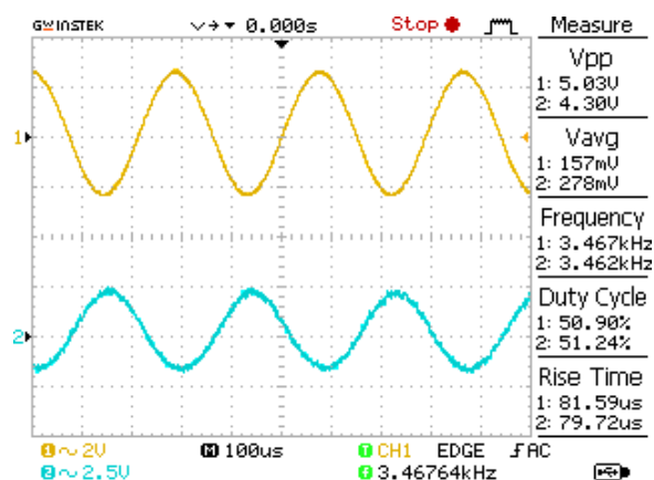
■ Gambar 17. Sinyal Pengukuran dengan Filter Warna Kuning
