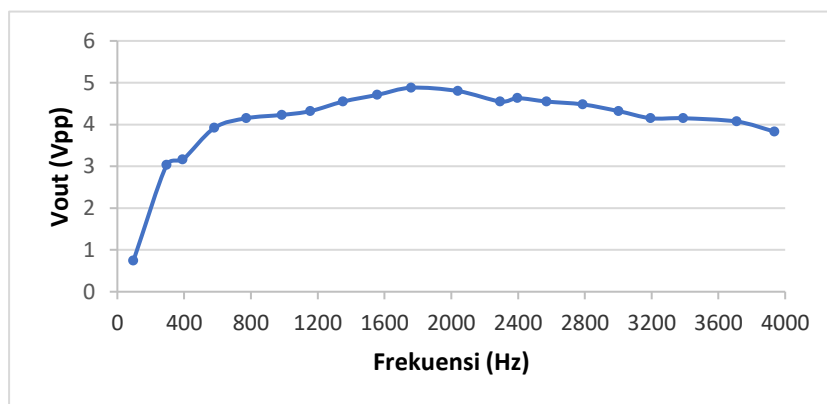
■ Gambar 21. Grafik Pengukuran dengan Filter Warna Hijau
