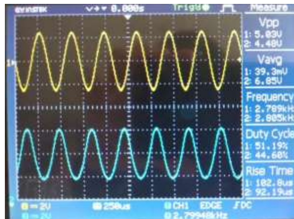
■ Gambar 20. Sinyal Pengukuran dengan Filter Warna Hijau
