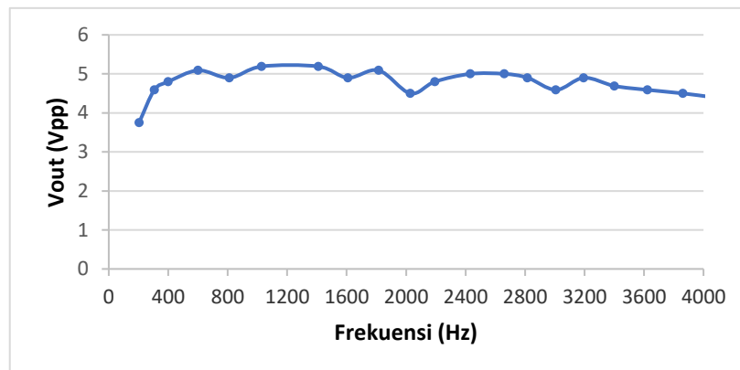
■ Gambar 12. Grafik Pengukuran Sistem tanpa Filter
