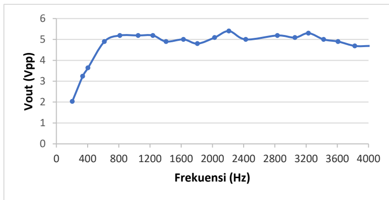
■ Gambar 15. Grafik Pengukuran dengan Filter Warna Merah
