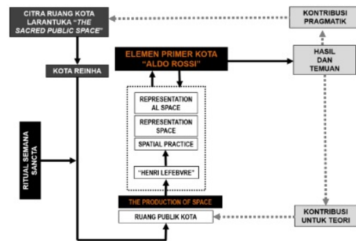
Gambar 4. Kerangka penelitian
