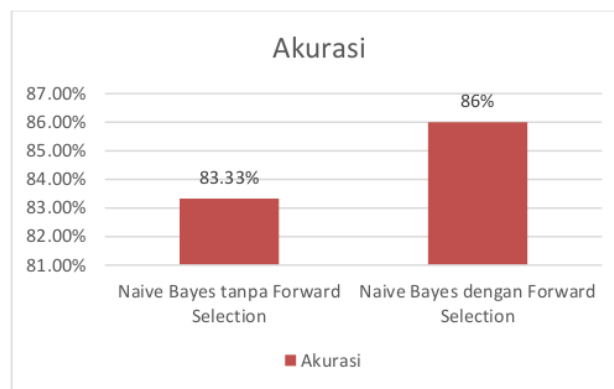
Gambar 3. Chart Perbandingan Hasil Akurasi
