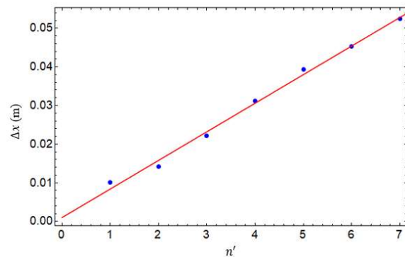
Gambar 5 Grafik perhitungan panjang gelombang sinar laser He-Ne
