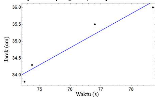
Gambar 3 Grafik perhitungan kelajuan sensor
