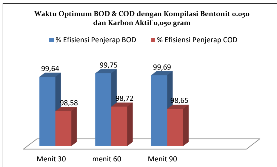
Gambar 1. Waktu Optimum Penjerapan BOD & COD Pada Limbah Cair Pabrik Karet
