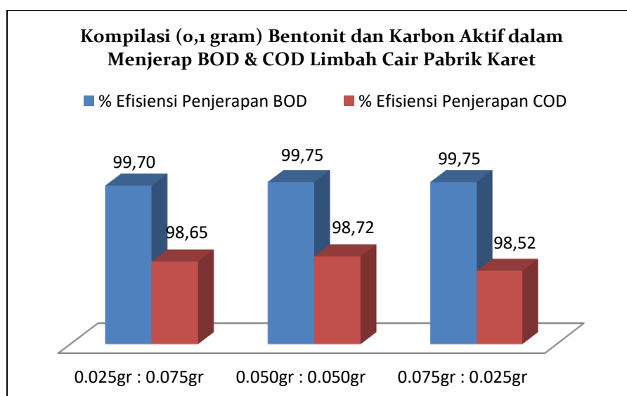
Gambar 2. Kompilasi Bentonit dan Karbon aktif dalam Menjerap BOD & COD Pada Limbah Cair Pabrik Karet
