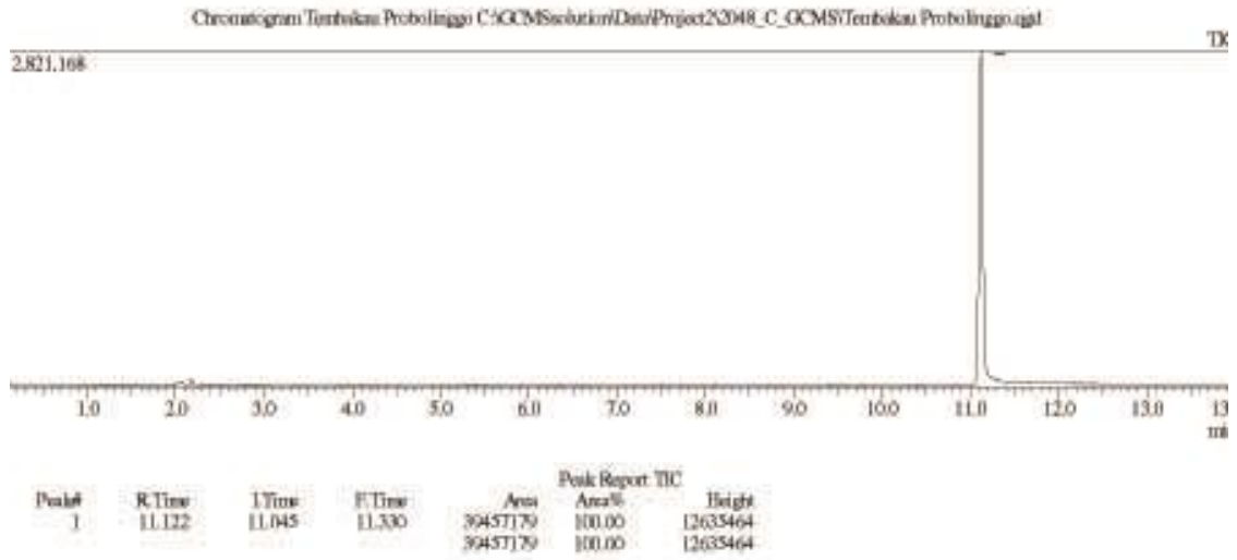
Gambar 6. Kromatogram GCMS Minyak Atsiri Tembakau Probolinggo
