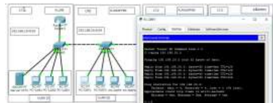
Gambar 5. Tes Ping 4
