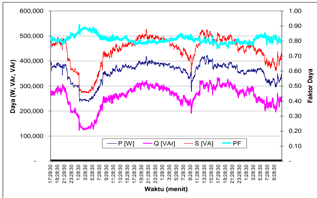
Gbr. 11 Konsumsi daya listrik di Pabrik Setempat 28 -30 Oktober 2008, pabrik teh 'studi'
