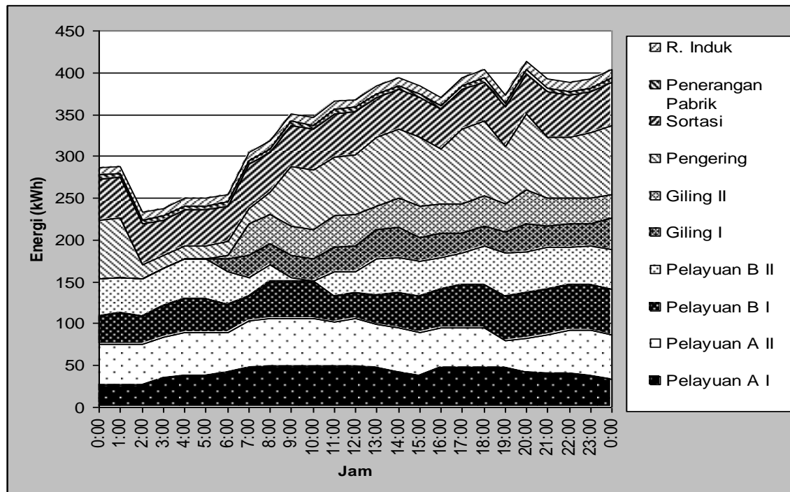
Gbr 9. Profil pemakaian energi proses selama 24 jam pabrik teh ‘studi’
