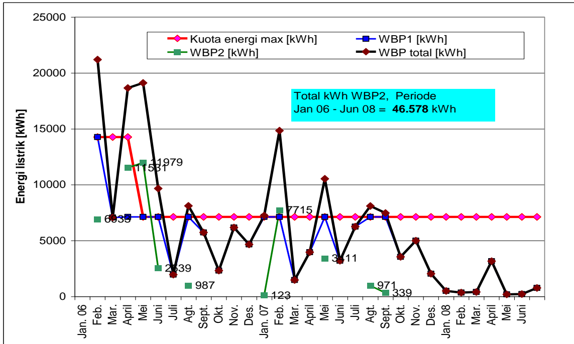
Gbr 7. WBP pabrik teh 'studi', Jan. 2006 – Juni 2008
