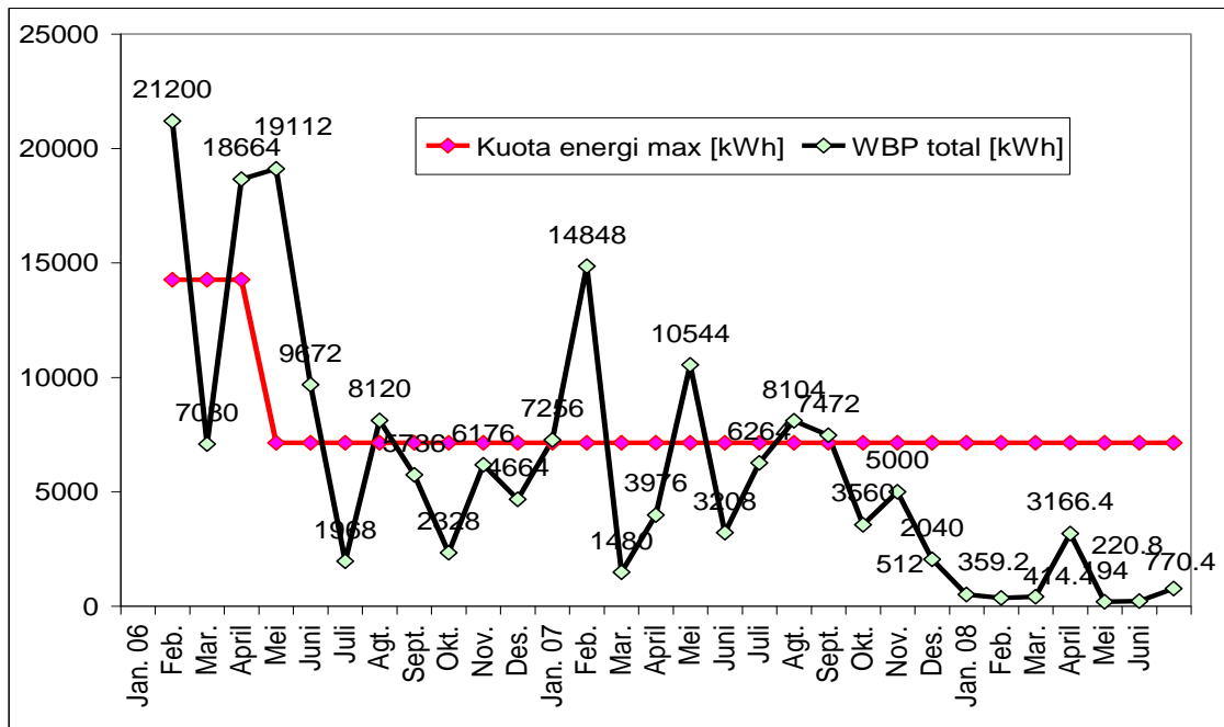
Gbr 6. Kuota energi max dan WBP total pabrik teh 'studi', Jan. 2006 – Juni 2008
