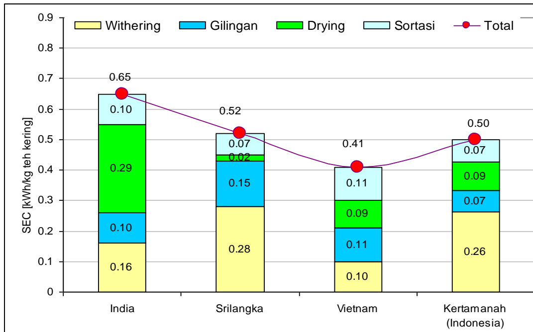
Gbr 15. Perbandingan nilai SEC Pabrik 'studi' dengan pabrik teh di berbagai negara
