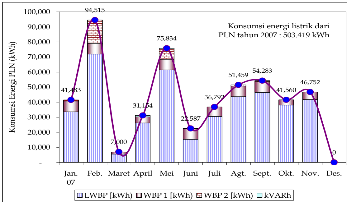
Gbr 4. Pemakaian energi listrik bulanan pabrik teh 'studi' tahun 2007
