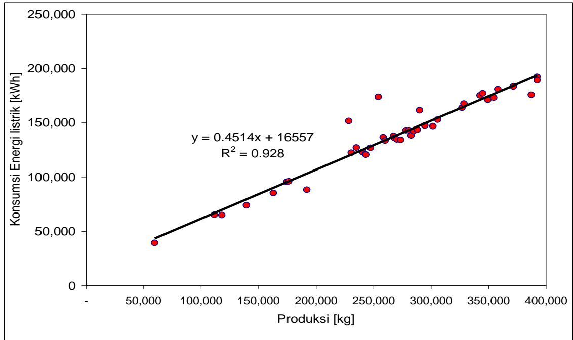
Gbr 13. Hubungan konsumsi energi vs produksi teh, setempat 28 -30 Oktober 2008
