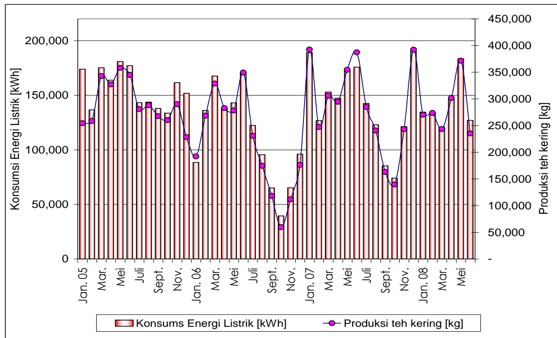
Gbr 12. Konsumsi energi vs produksi teh, setempat 28 -30 Oktober 2008
