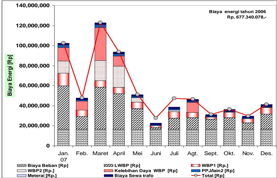
Gbr 3. Biaya energi listrik bulanan pabrik teh 'studi' tahun 2006
