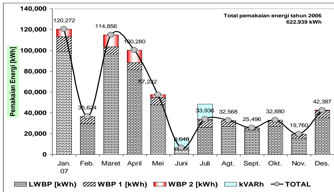
Gbr 2. Grafik pemakaian energi listrik bulanan pabrik teh 'studi' tahun 2006
