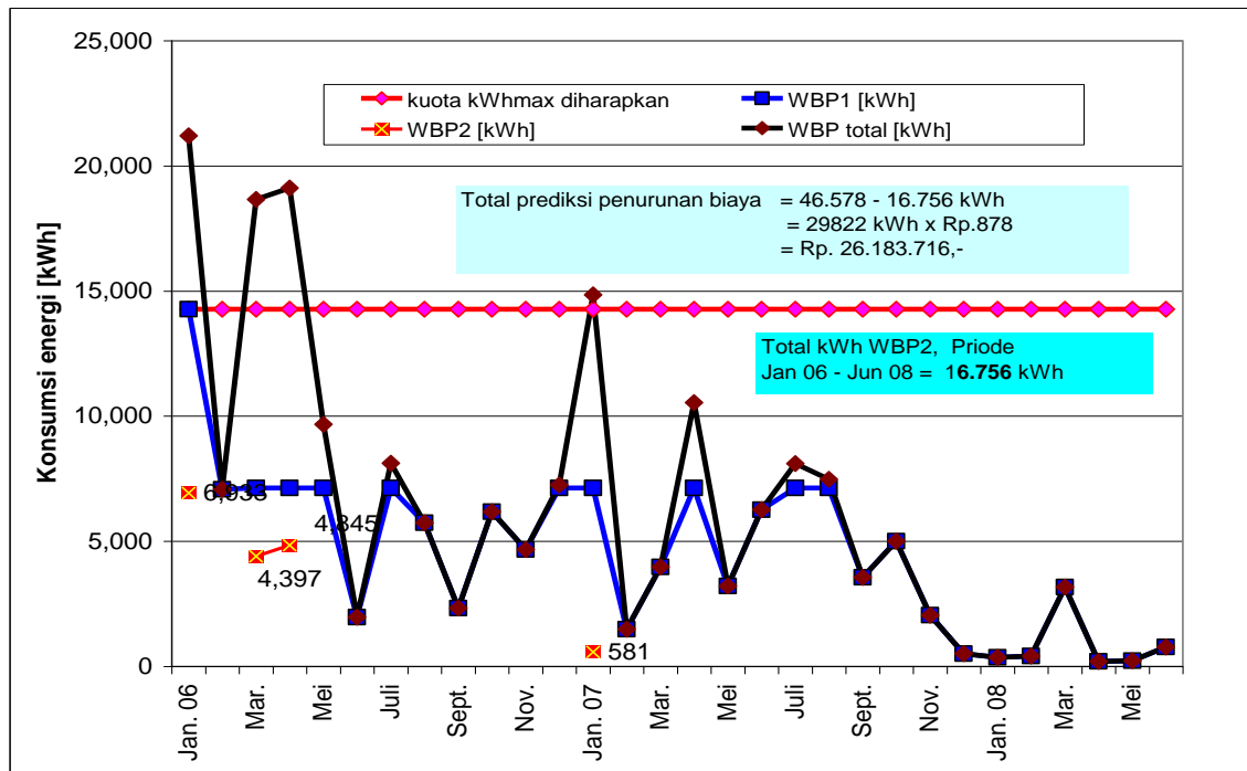
Gbr 8. WBP pabrik teh 'studi', Jan. 2006 – Juni 2008
