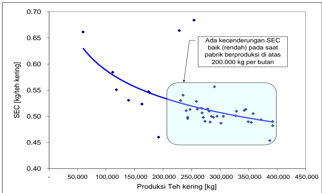
Gbr 14. Hubungan SEC vs produksi teh, setempat 28 -30 Oktober 2008
