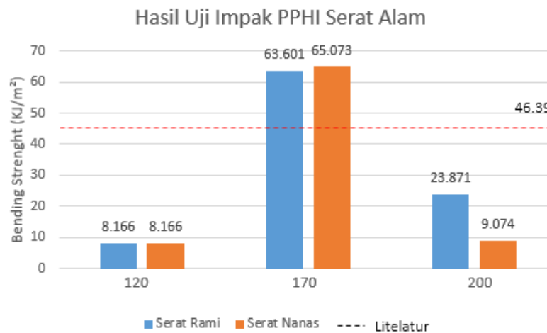
Gambar 8. Grafik Hasil Uji Impak PPHI Serat Alam
