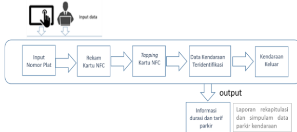
Gambar 6. Gambaran Umum Alur Sistem Parkir
