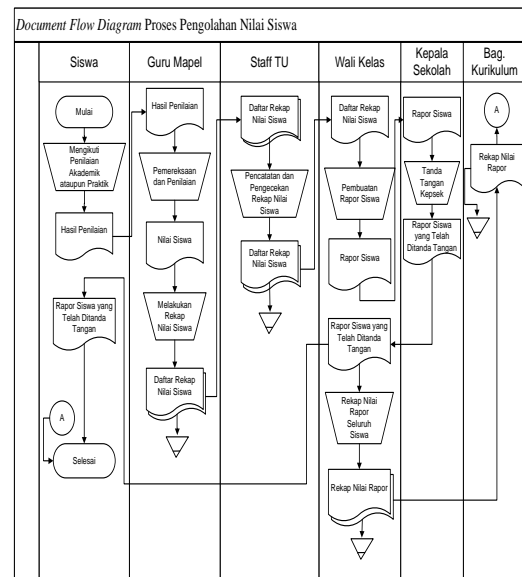
Gambar 1 Dokument Flow Diagram Pengolahan Nilai Siswa
