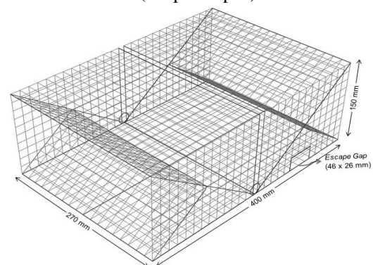
Gambar 5. Desain bubu dengan escape gap (tampak keseluruhan)
