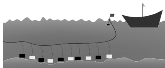
Gambar 1. Ilustrasi penyusunan bubu (bubu terang: bubu dengan escape gap , bubu gelap: bubu tanpa escape gap )
