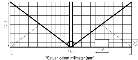
Gambar 4. Desain bubu dengan escape gap (tampak depan)
