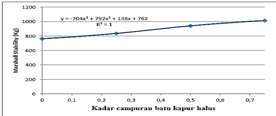
Gambar 7. Grafik Nilai Stabilitas.
