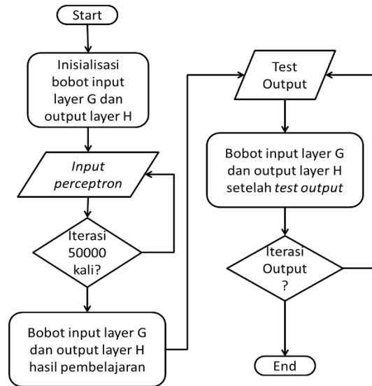
Gbr. 3. Diagram alir dari simulasi JST HEKM
