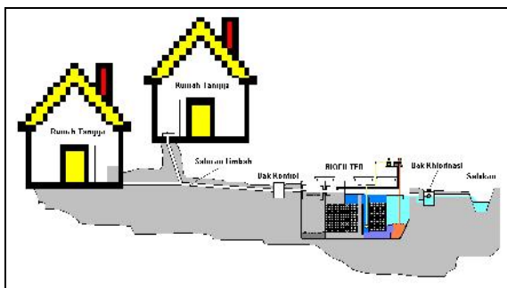
Gambar 8 : Bagan aliran air limbah dan proses pengolahan yang digunakan untuk percobaan.
