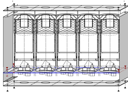
Gambar 1. Pencacahan 5 buah detektor dan 5 buah sampel/cuplikan
