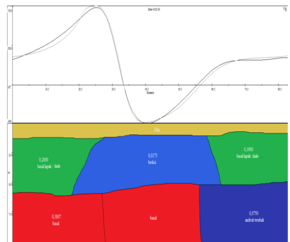
Gambar 11. Model Penampang Magnetik batuan pada lintasan A-A'
