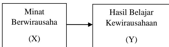
Gambar 1. Kerangka Berfikir
